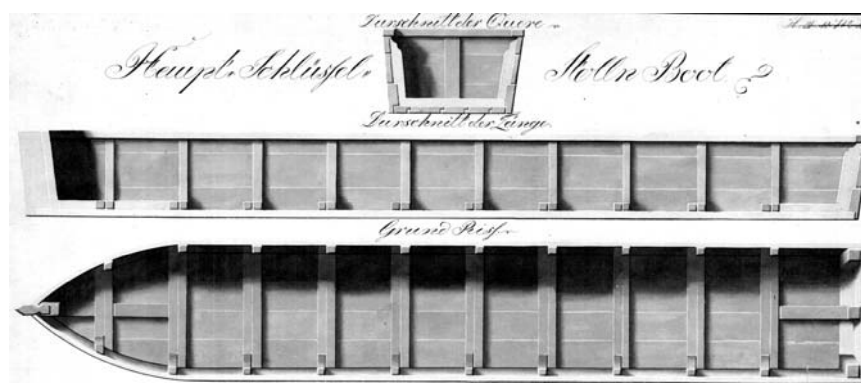
Rys. 9. Łódź do transportu skrzyń z węglem w sztolni
