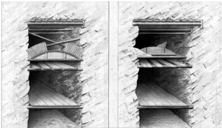
Rys. 5. Wykonywanie obudowy ostatecznej sztolni
